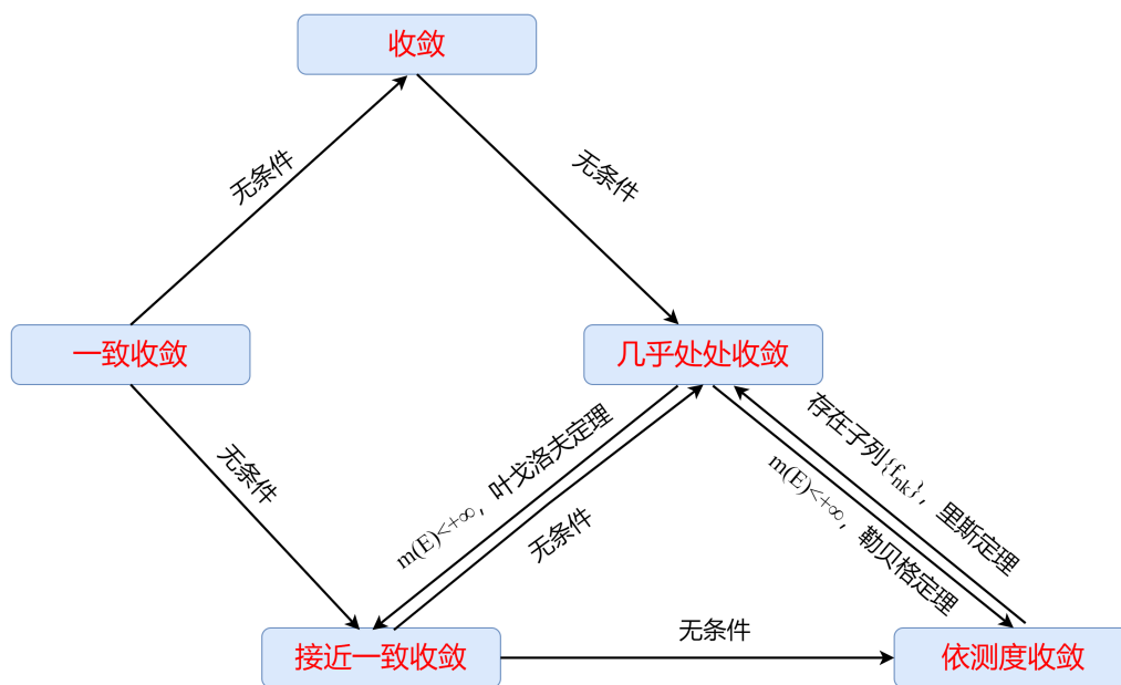
图 1: 几种收敛性之间的关系
